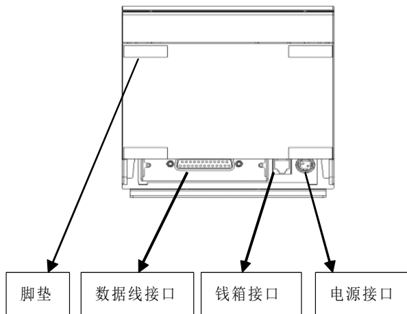
图 1：T90 背面图
