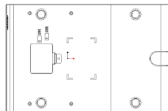
图 4：T90 底面图
